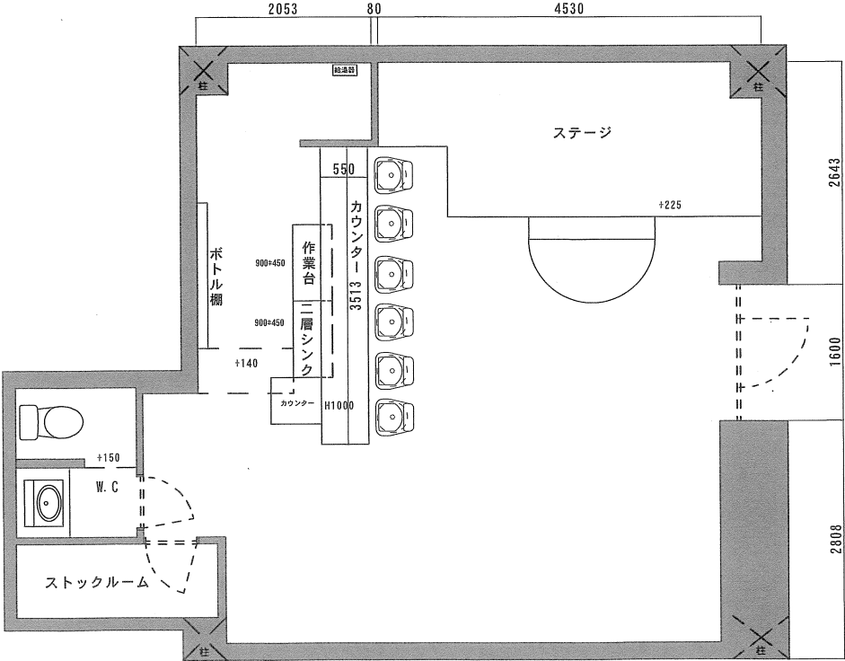
店舗平面図
